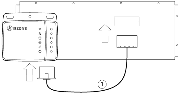
Anschlusschema
